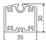
BUNNLIST BD 30
